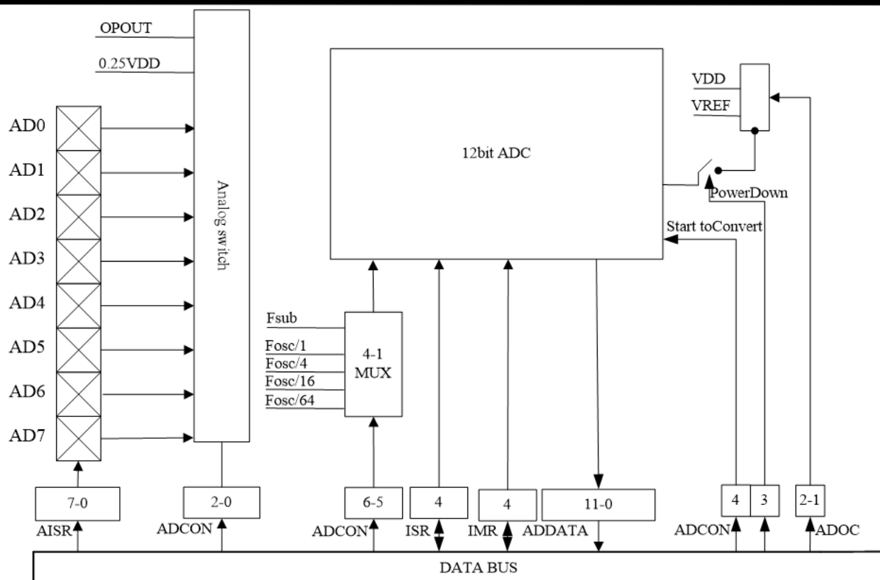
图 3 ADC 功能图
