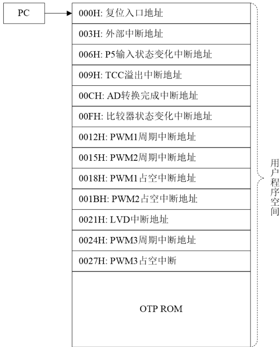
程序存储器结构
