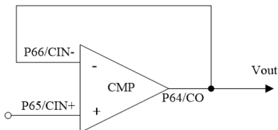
图 6 比较器输入选择 VREF
