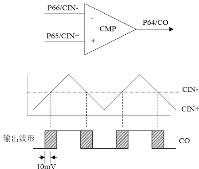
图 4 比较器功能图
