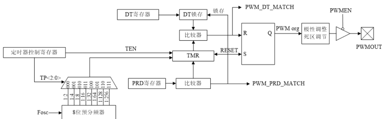
图2 PWM功能图
