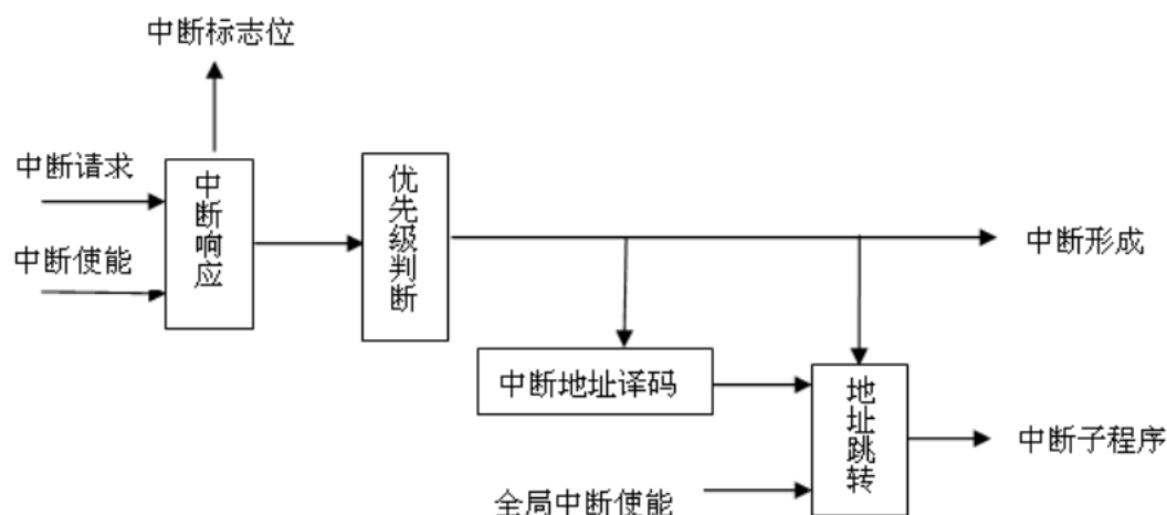
图 7 中断原理图
