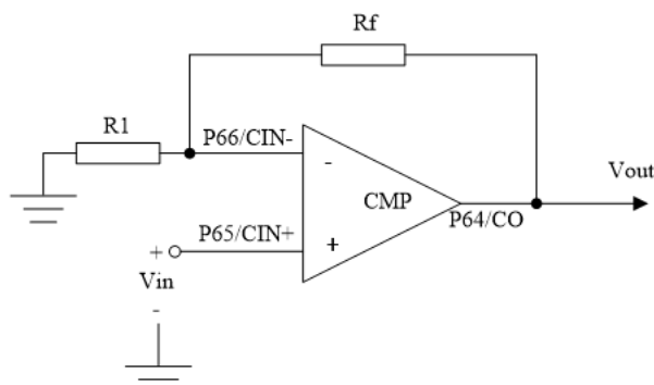
图 5 比较器用作 OP
